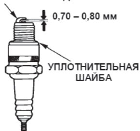
БОКОВОЙ ЭЛЕКТРОД
