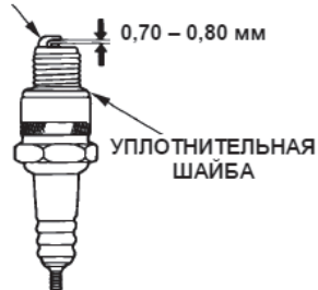
БОКОВОЙ ЭЛЕКТРОД
